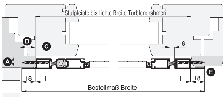
Horizontalschnitt
