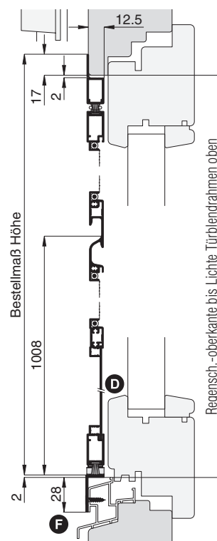
Vertikalschnitt
